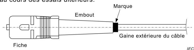
Figure B.1 – Marquage initial de la gaine du câble
