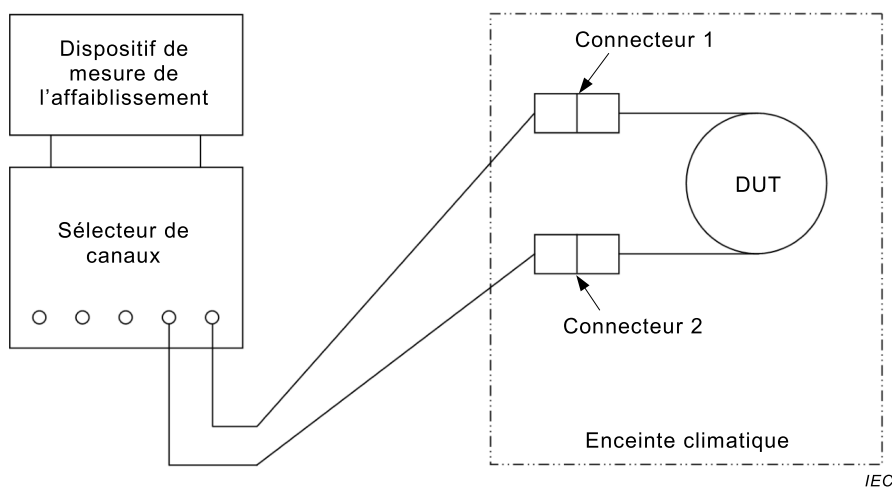
Figure C.1 – Configuration de l'essai de variations de température
